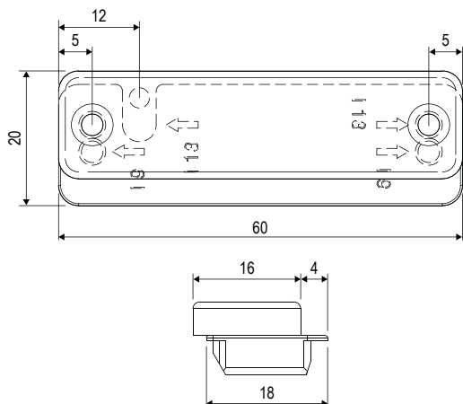
Posizionamento reed in asse 13
