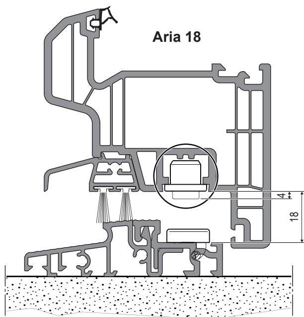
Applicazione con magnete da fissare con vite e spessore compensatore per canalino 16/12 A48902.19.01
