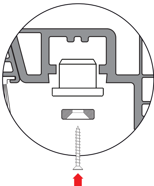
Applicazione con magnete da fissare con vite e spessore compensatore per canalino 16/12 A48902.19.01
