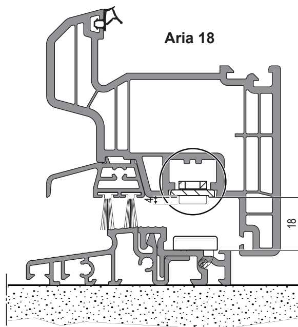
Applicazione con magnete da fissare con vite alla ferramenta.
