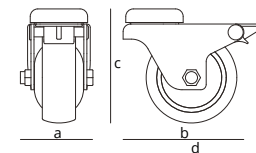
SUPPORTO GIREVOLE | REVOLVING BODY
