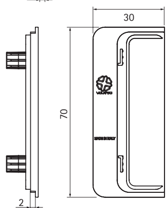
Tappo terminale esterno lavastoviglie Dishwasher external caps
