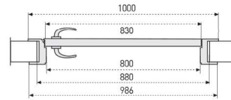
Scorrevole listellare Blockboard sliding door
