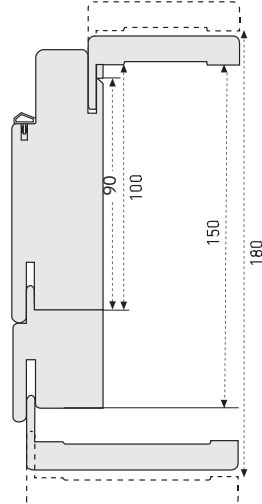
Telaio con ringrosso fino a 180 mm
