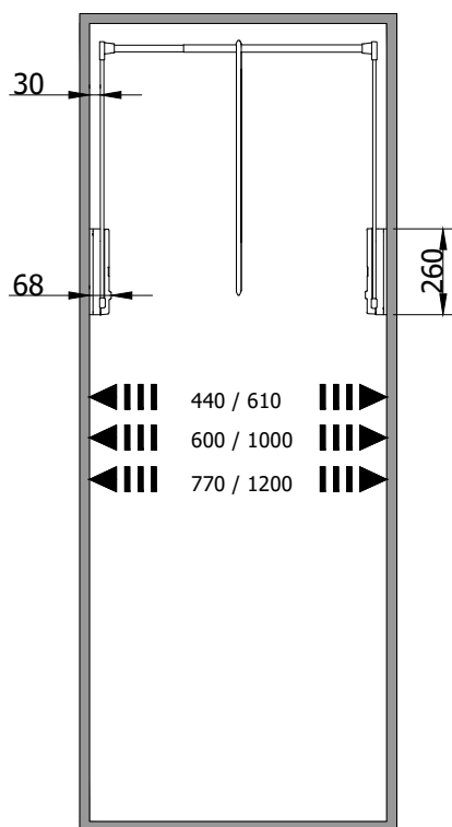
NERO - TUBO GRIGIO black - grey tube
