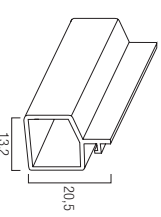
Terminale Pvc Super TERPV/CPA 13,2 x 20,5 mm
