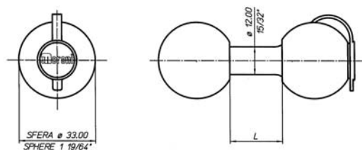
Luccotto rivestito con tappo antipolvere Plastic covered "luccotto" with dust cover
