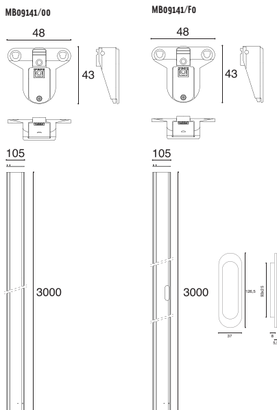
Vista retro (per versione anta scorrevole verticale)
