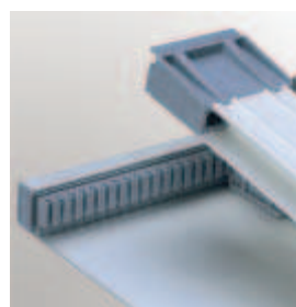
la foto mostra l'applicazione dello spingitoio sulla cremagliera
