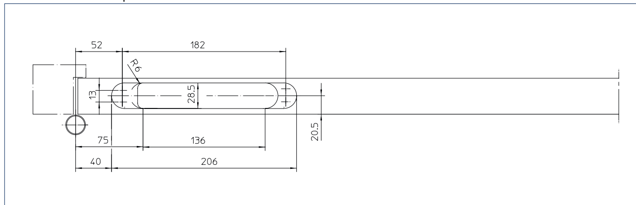
Lavorazione su anta complanare
