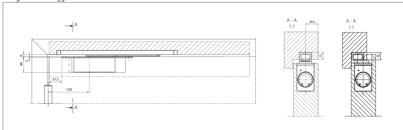
Disegno di montaggio
