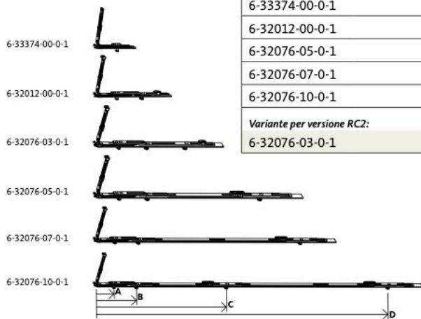
Chiusure inferiori DK per anta ribalta - serie 6-32076 - campo d'applicazione
