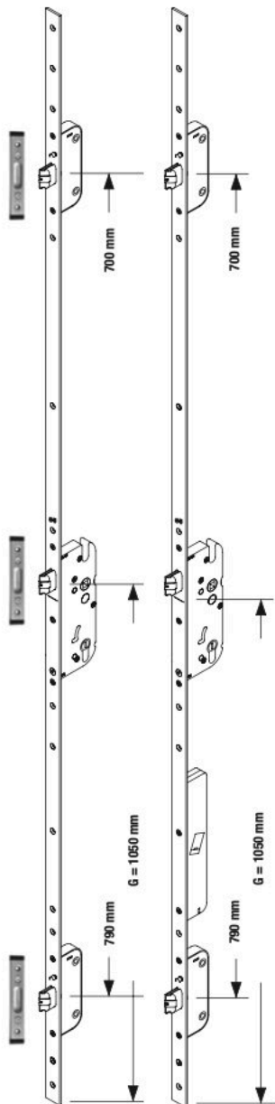
Disegno tecnic 1 anta Legno 0-44427-LO
