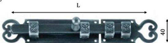
Art. 2118/ Catenaccio Traverso Orizzontale Bolt
