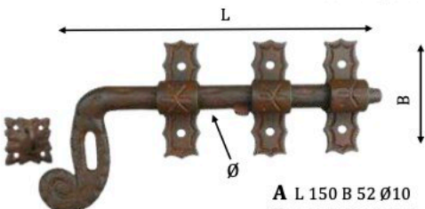
Art. 1021/ Catenaccio portallucchetto Aldrop bolt
