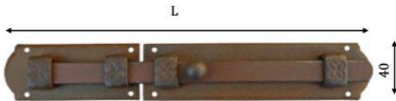
Art. 1892/ Catenaccio Traverso Orizzontale Bolt
