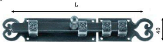
Art. 1894 Catenaccio Traverso 115x40mm Orizzontale Bolt 115x40mm
