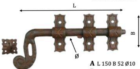
Art. 1021/ Catenaccio portalucchetto Aldrop bolt
