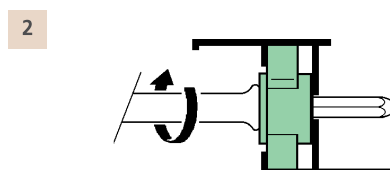
2 Calettamento a scatto per rotazione Agire in senso orario mantenendo il RAPID-BLOCK aderente al serramento
