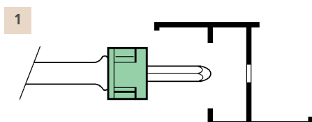
1 Inserimento frontale Appoggiare il "grano filettato" sul risalto di contrasto della chiave
