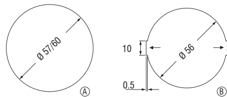
Foro di incasso / Recessed hole / Einbaumaße
