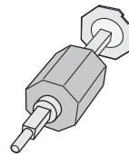
2200026 Fondello regolabile in materiale plastico con perno tondo per tubo ottagonale Ø70 Adjustable plastic cap with pivot for Ø70 octagonal rolling tube
