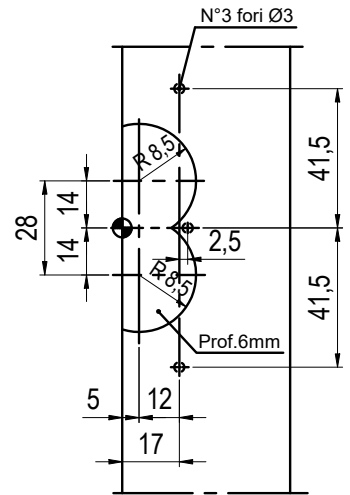
ARIA 12-BATTUTA 18 INTERASSE 9 e 13
