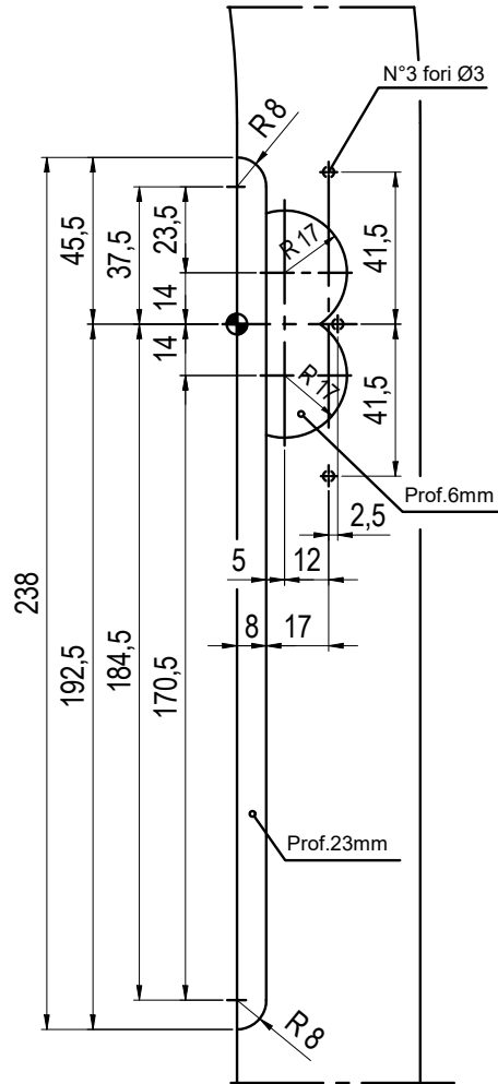
ARIA 4-BATTUTA 18 INTERASSE 13
