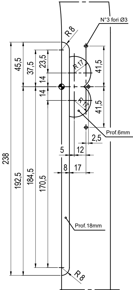
ARIA 4-BATTUTA 18 INTERASSE 9
