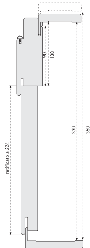
Telaio con foglio bussola fino a 350 mm
