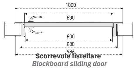
Sezione orizzontale Horizontal section
