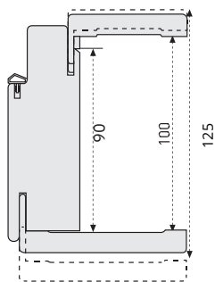
Telaio con coprifilo aletta lunga fino a 140 mm
