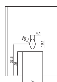
LAVORAZIONE MACHINING
