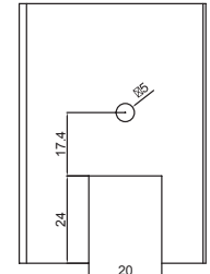
LAVORAZIONE MACHINING
