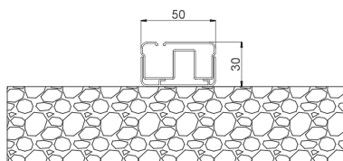
orizzontale foro
