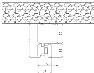
verticale foro
