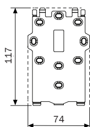
Staffa di fissaggio
