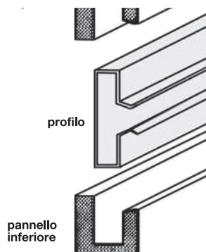
montaggio dei pannelli in sovrapposizione
