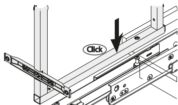
montaggio della guida inferiore
